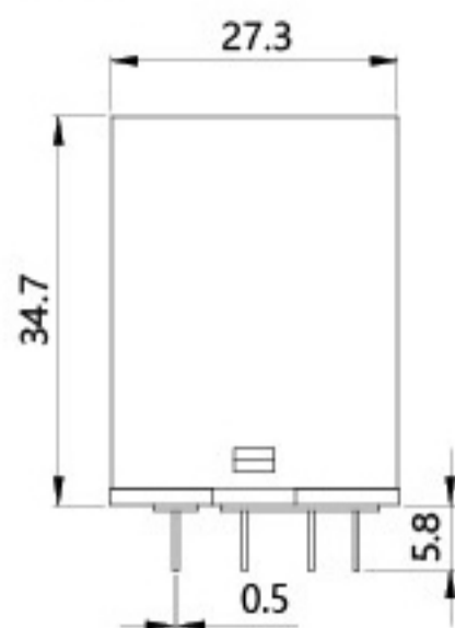
正面图
