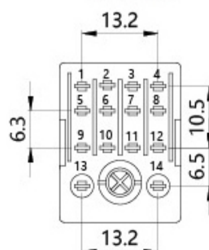
安装尺寸
