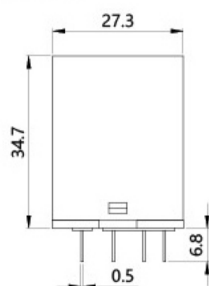
正面图
